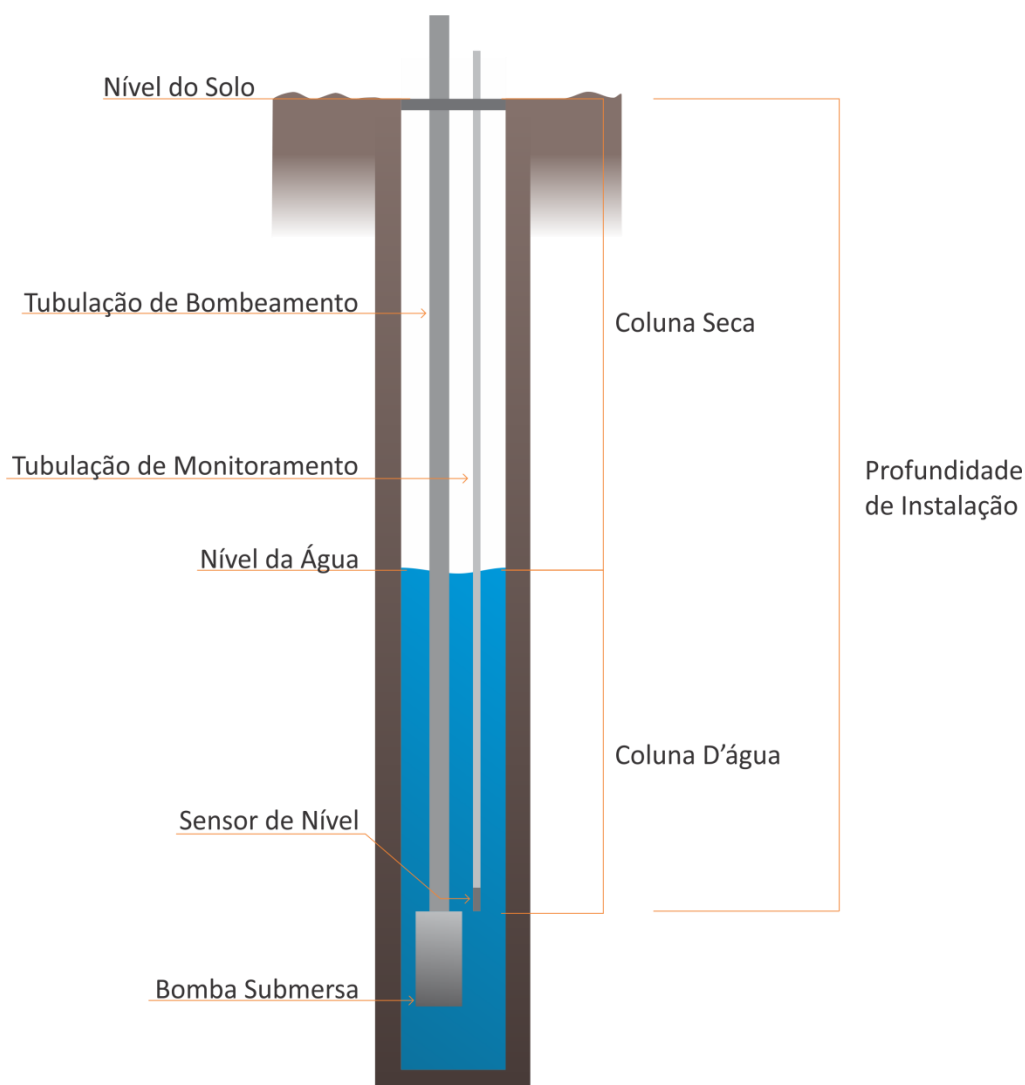
Figura 2 – Diagrama de instalação do sensor de nível.
