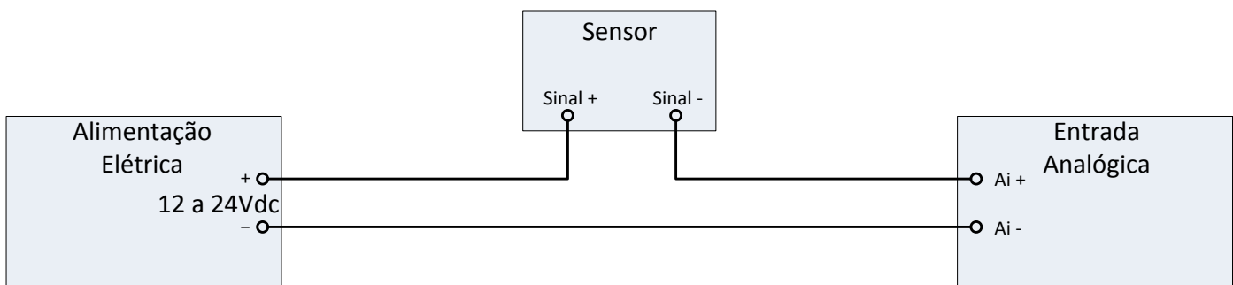
Figura 1 – Ligação do sensor de nível ao Hidrobox
